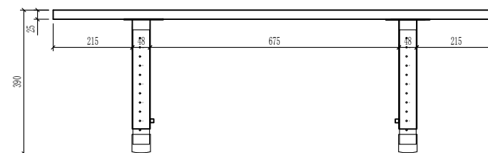
Round Table - 120 x 120cm 39-61.5cm
